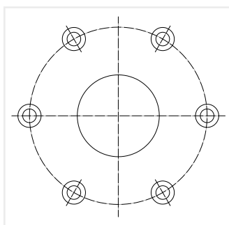
Gatenplannen 6M247
