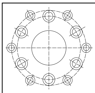
Gatenplannen 12M255
